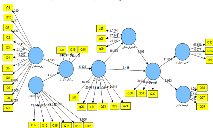
شکل ۲. مقدار تخمین زده شده هریک از ضرایب مسیر
